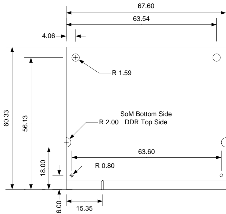
SoM SODIMM 200 Module Dimensions
