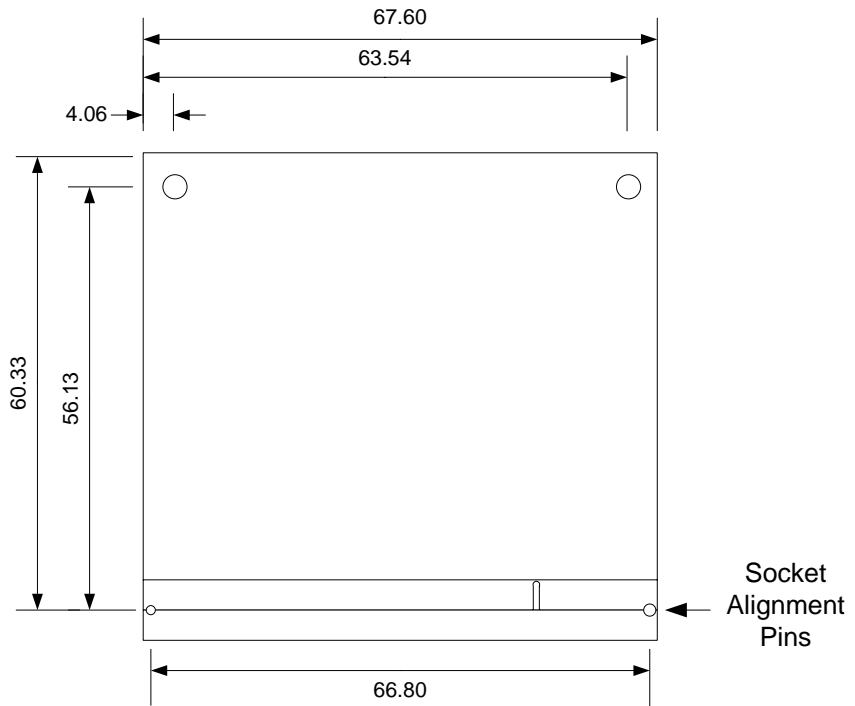
SoM SODIMM 200 Carrier Dimensions
